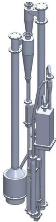
Fig. 8. Chalmers 100 kW unit.
